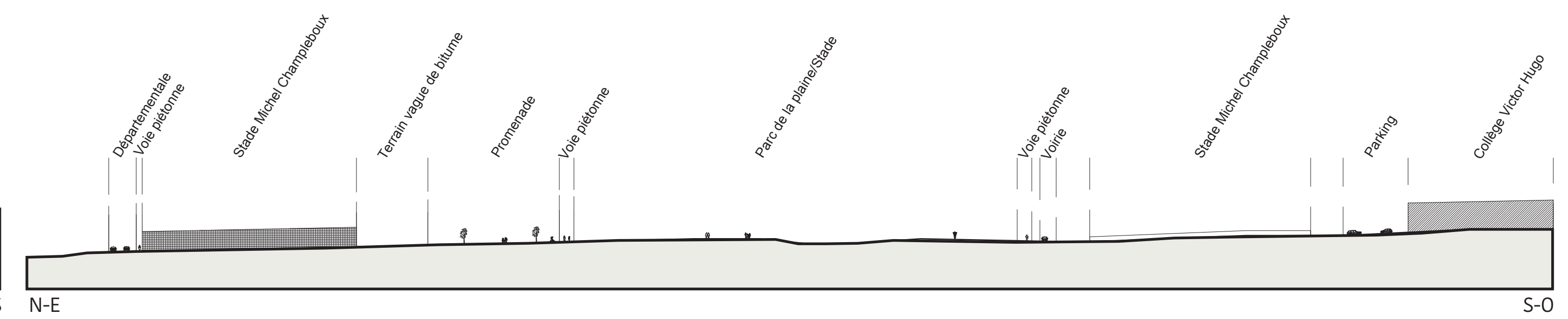
Coupe longitudinale de l'existant BB'
